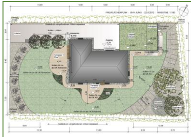
Freiflächenplan
