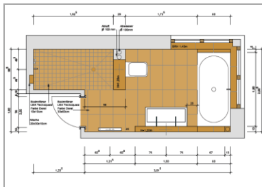
Badplanung
