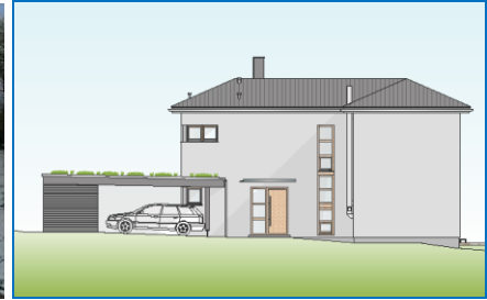
Neubau Wohnhaus in Holz (KfW Effizienzhaus 55)
